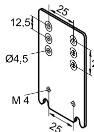
Uchwyt rurki kapilarnej do kontrolerów szronu standardowy Nr części: 803 778
