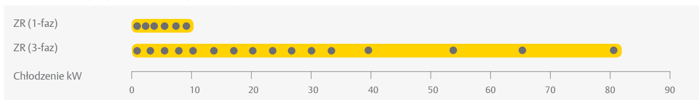
Sprężarka spiralna ZR
