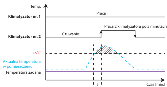
schemat pracy 2 klimatyzatorów w funkcji kaskady
